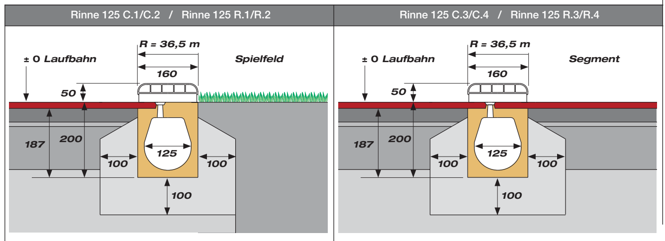
ANRIN SPORT Entwässerungssystem 125 Schlitzrinne Rinne 125 C.1/C.2 Rinne 125 R.1/R.2
